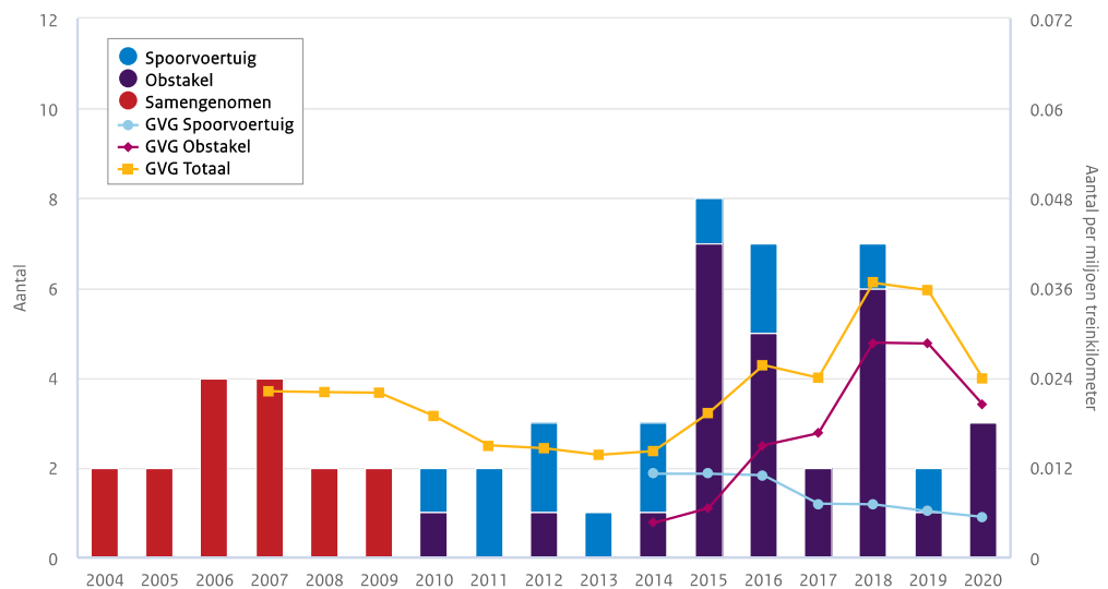
Figuur C.1: Trend in het aantal significante botsingen en de bijbehorende GVG's over de jaren 2004-2020. Pas vanaf 2012 zijn botsingen met obstakels, zoals stootbuffers, apart geregistreerd. Voor 2010 en 2011 is dit onderscheid retrospectief aangebracht, om een apart GVG spoorvoertuig en GVG obstakel vanaf 2014 beschikbaar te hebben. Pas vanaf 2015 zijn botsingen met de bovenleiding geïncorporeerd. Bron: ILT .
