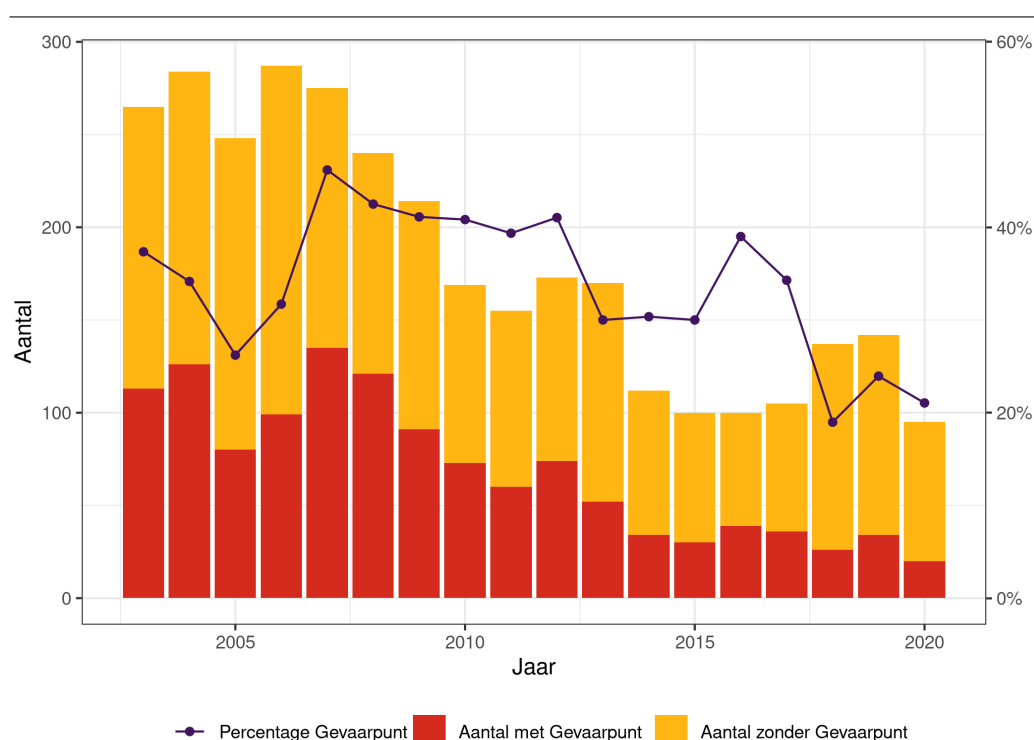
Figuur F.2: Trend in het aantal STS -passages met gevaarpunt over de jaren 2003-2020. Het gestapelde staafdiagram geeft de aantallen weer ten opzichte van de linker as. De groene trendlijn laat het percentage STS -passages met gevaarpunt zien ten opzichte van de rechter as. Bronnen: ProRail en ILT .
