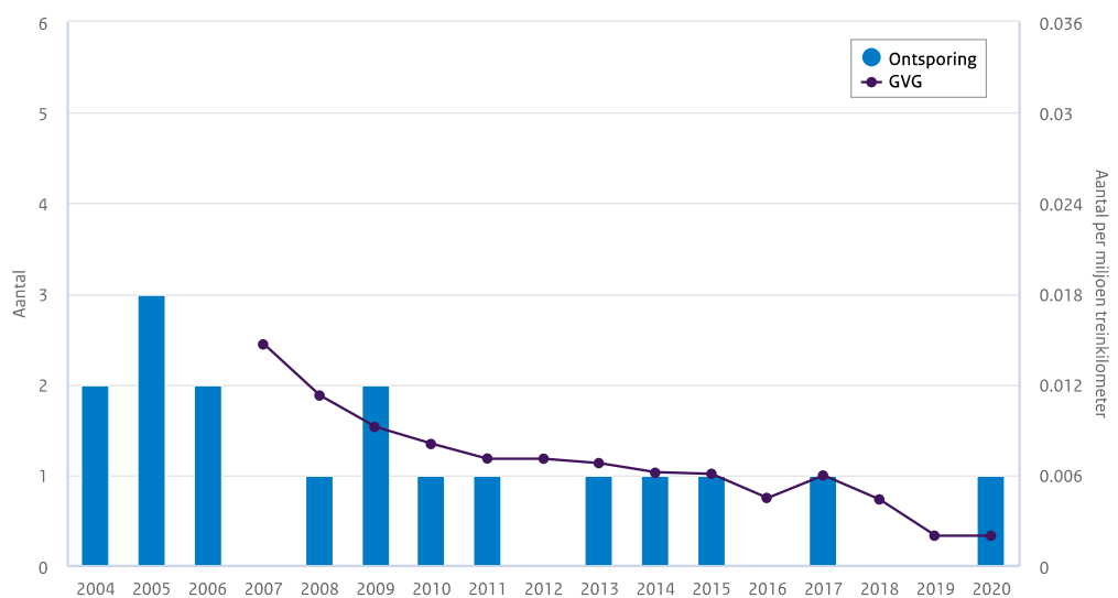
Figuur C.2: Trend in het aantal significante ontsporingen en het bijbehorende GVG over de jaren 2004-2020. Bron: ILT .
