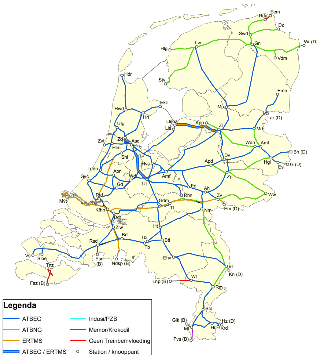
Figuur A.2: Overzichtskaat van de treinbeïnvloedingssystemen op het hoofdspoor (Situatie januari 2018). Uit: ProRail Netverklaring 2018, Bijlage 14.
